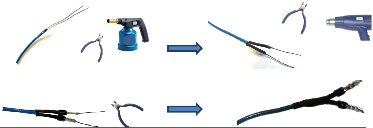
A la flamme enlever la matière d'isolation et la matière noire du cuivre. Appliquer les gaines thermo rétractables et les rétreindre à l'air chaud.
