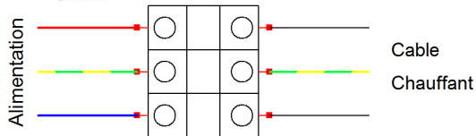
Boîte de raccordement électrique pour B100 et M100 :
